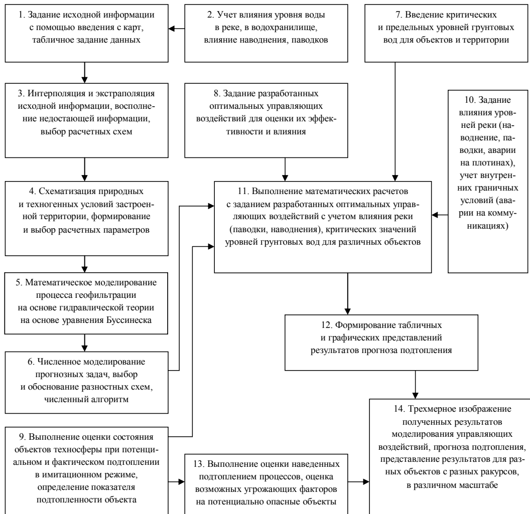
Рисунок 2 – Процессуальная схема решаемых задач на ПДСОМ для выполнения оценочных прогнозов подтопления и наведенных опасных природных процессов
