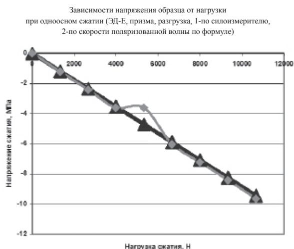
Рис. 5. Экспериментальная и ультразвуковая зависимости напряжения при разгрузке (ЭД – 6)
