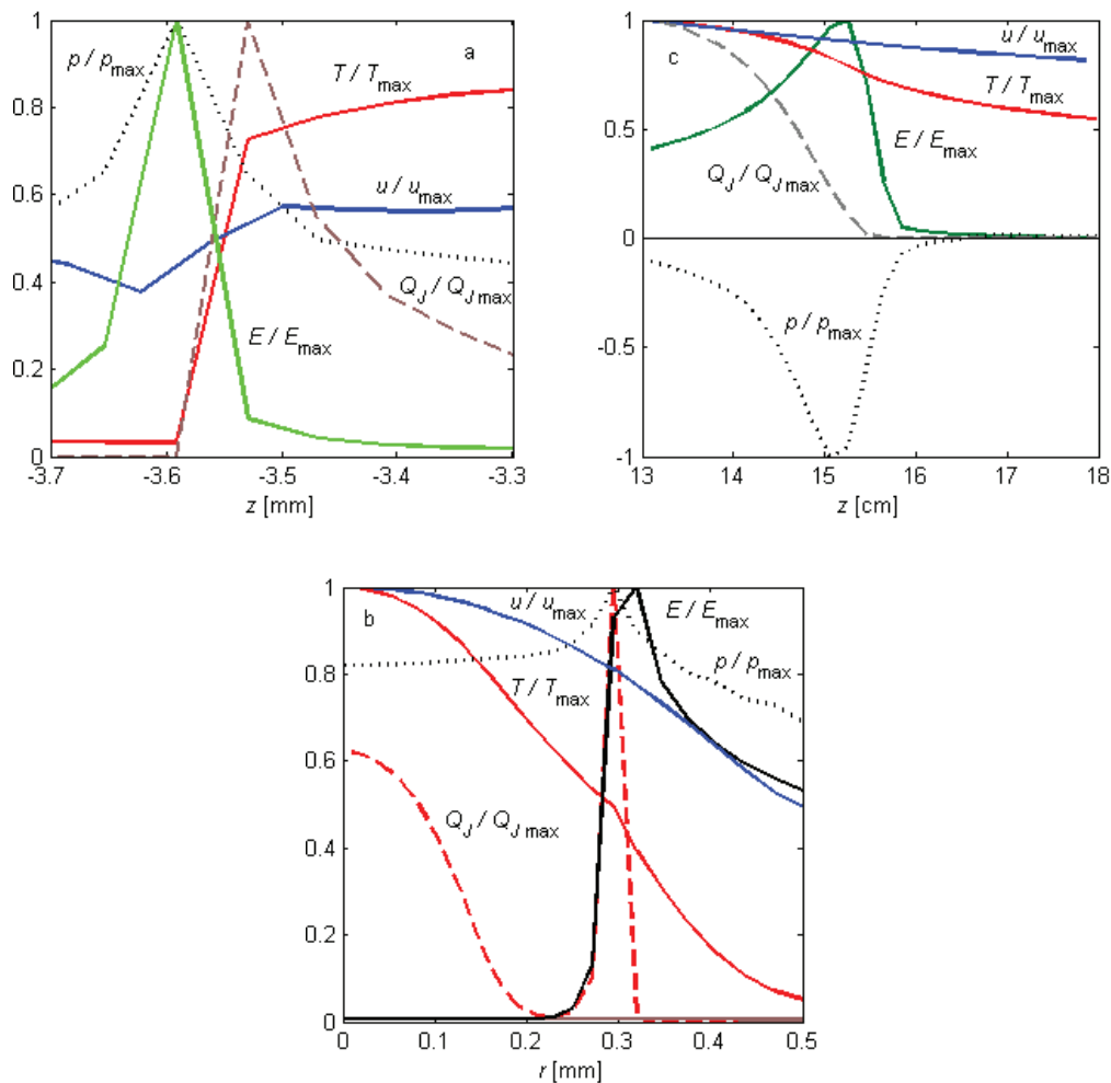
Рисунок 6 – Изменения характеристик (а,с; r = 0 ; б; z = 0 ) Q_n = 1000 Вт, G_0 = 5 л/мин
