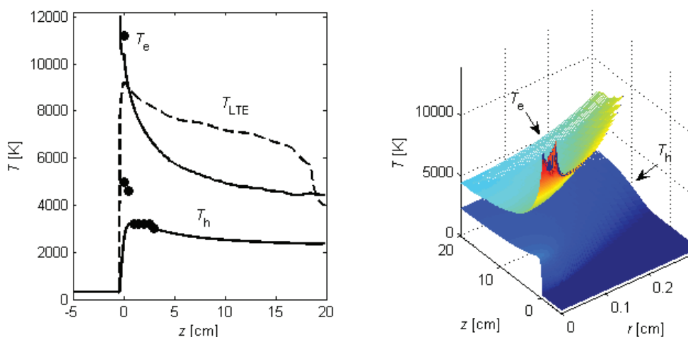
Рисунок 7 – Распределение температуры электронов T_e , тяжелых частиц T_h , (пунктир – равновесная модель T_{LTE} ; точки – эксперименты [7, 9, 10])
