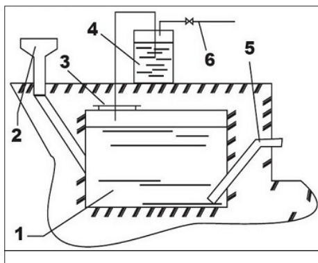
Рисунок 1 – Схема биогазовой установки малой мощности
