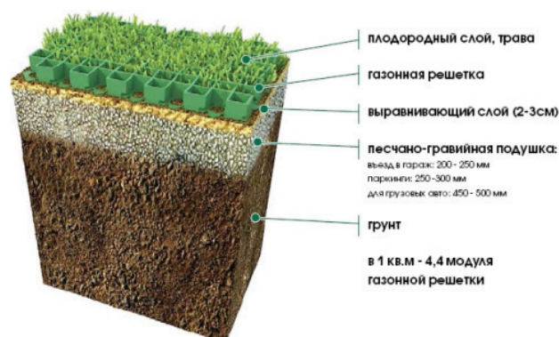
Рисунок 5 – Принципиальная схема конструкции газонной решетки экопарковки
