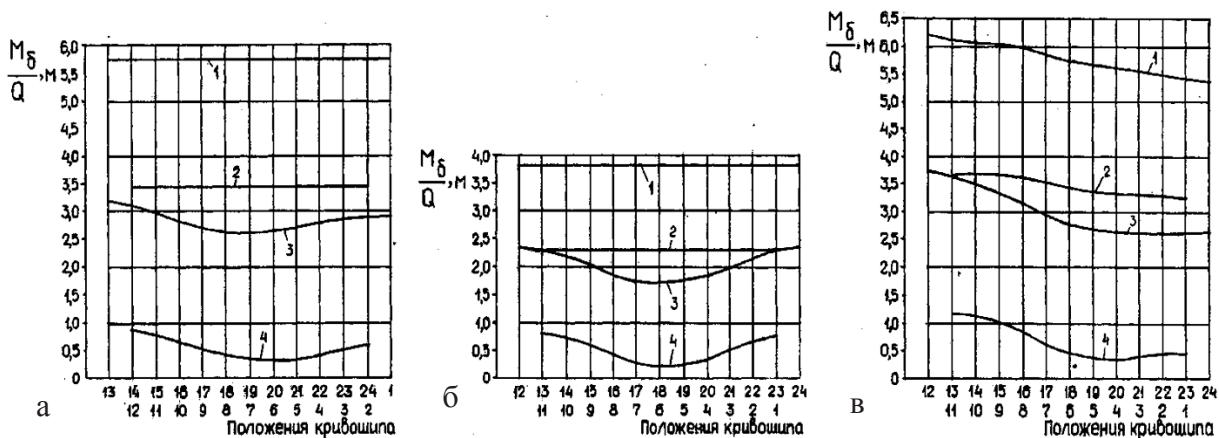
Рисунок 1 – Момент нагрузки на балансира при кривошипном (1, 2) и комбинированном (3, 4) уравнивании; (1, 3) – при рабочем и (2, 4) – при холостом ходе
