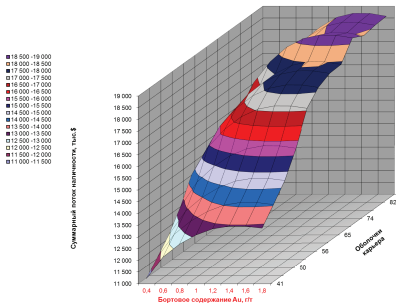
Рисунок 2 – Скрин 3D-модели результатов совместной оптимизации оболочек карьера и бортового содержания [3]
