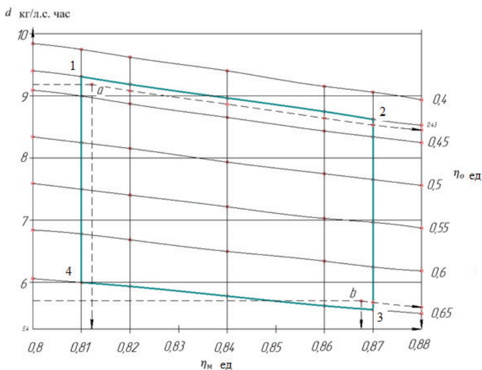
Рисунок 2 – Семейство кривых удельных расходов пара от механического \eta_m и относительного индикаторного \eta_{oi} , КПД
