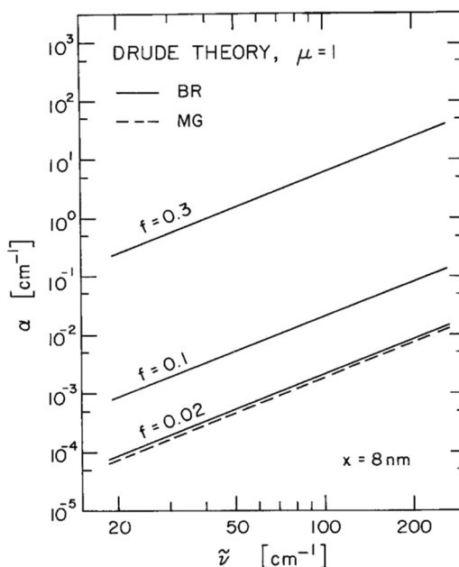
Рисунок 3 – Коэффициент поглощения \alpha среды с наночастицами алюминия диаметром 8 нм в зависимости от частоты для трех значений фактора заполнения f (из работы [11, с. 35]; подробности см. в [11])
